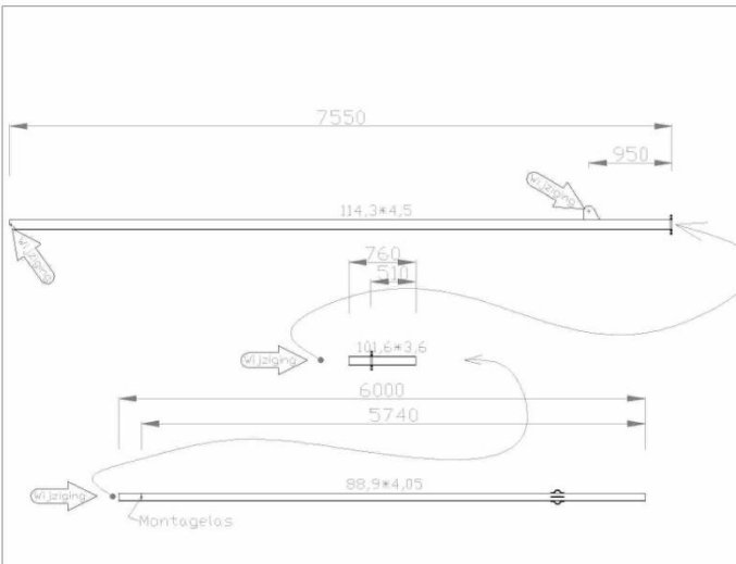
Schaal 1:20
