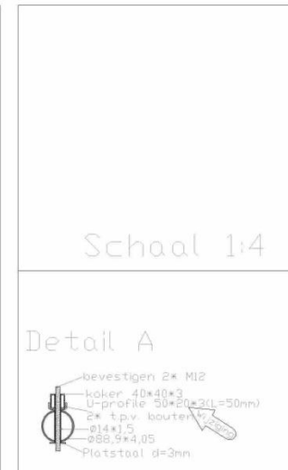
Schaal 1:4
